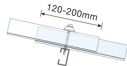
SOVRAPPOSIZIONE ELEMENTI Il sormonto minimo delle lastre TEGOLUX® sulla larghezza deve essere di 120mm.
