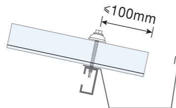
SPORGENZA ESTREMITÀ All'estremità della copertura le lastre non devono sporgere oltre la gronda più di 100mm.
