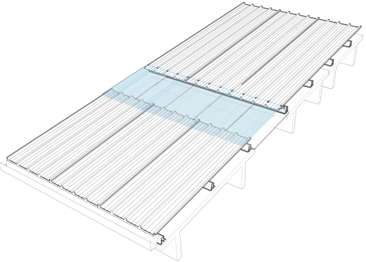
LUCERNARI TRASVERSALI Realizzazione di lucernari trasversali in accoppiamento con pannelli monolitici
