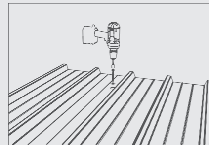
Foratura e fissaggio con avvitatore
