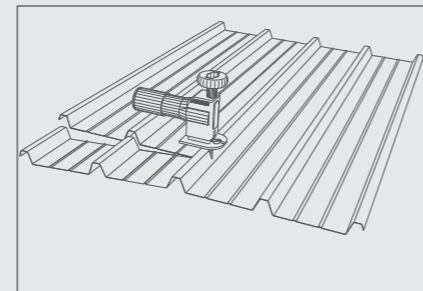
Taglio delle lastre con seghetto alternativo
